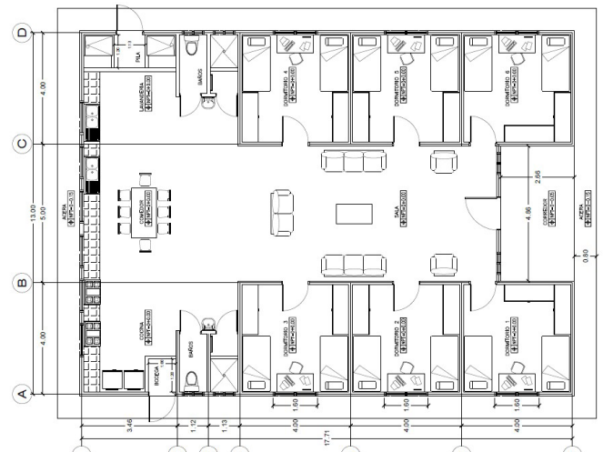
Der Grundriss des geplanten Schülerwohnheims für 24 Stipendiaten
